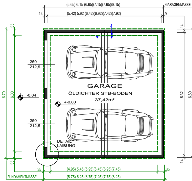
GRUNDRISS
