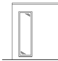
STREIFEN-FENSTER "STEHEND" B/H 60/200cm
