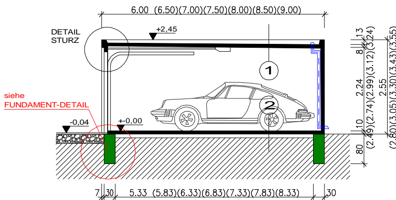
SCHNITT
