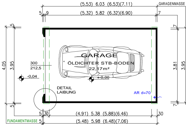
GRUNDRISS
