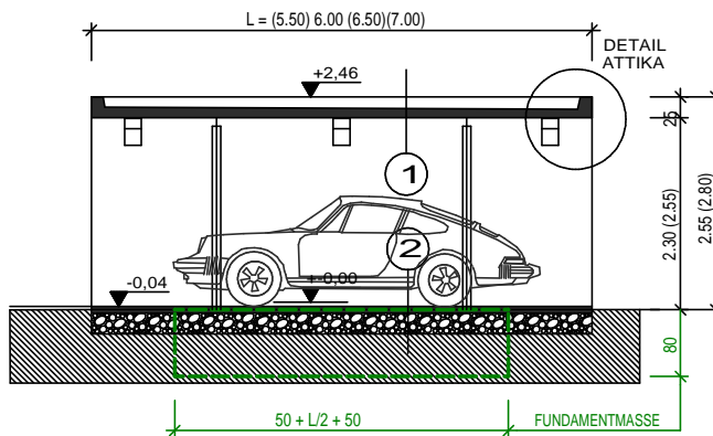
SCHNITT
