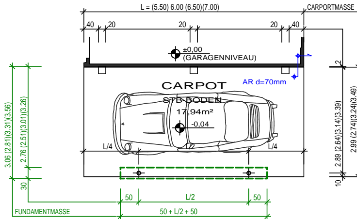
GRUNDRISS
