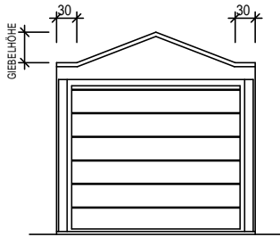
"DREIECKSGIEBEL" OHNE LOCH
