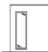
STREIFEN-FENSTER "STEHEND" B/H 60/200cm
