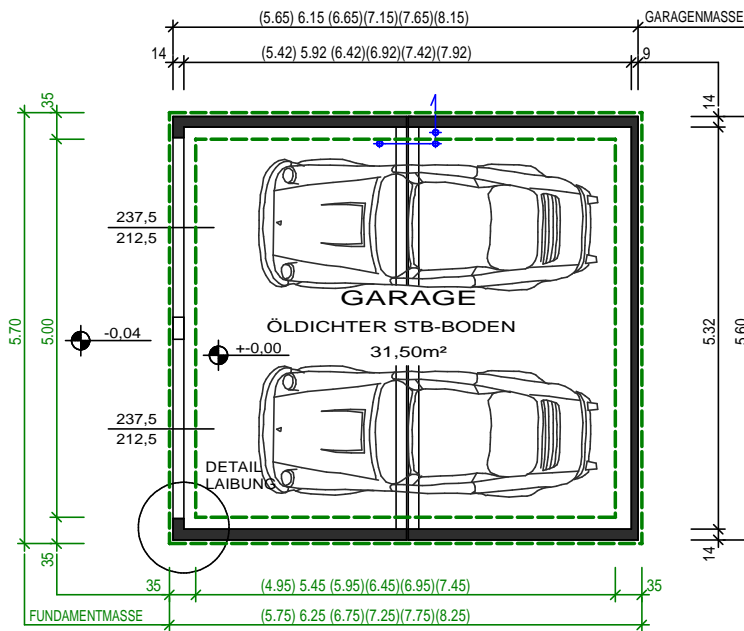
GRUNDRISS
