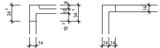
DETAIL STURZ
