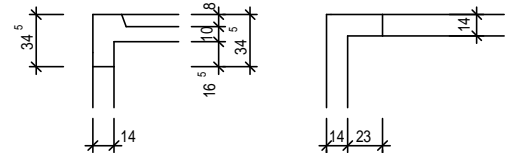
DETAIL STURZ
