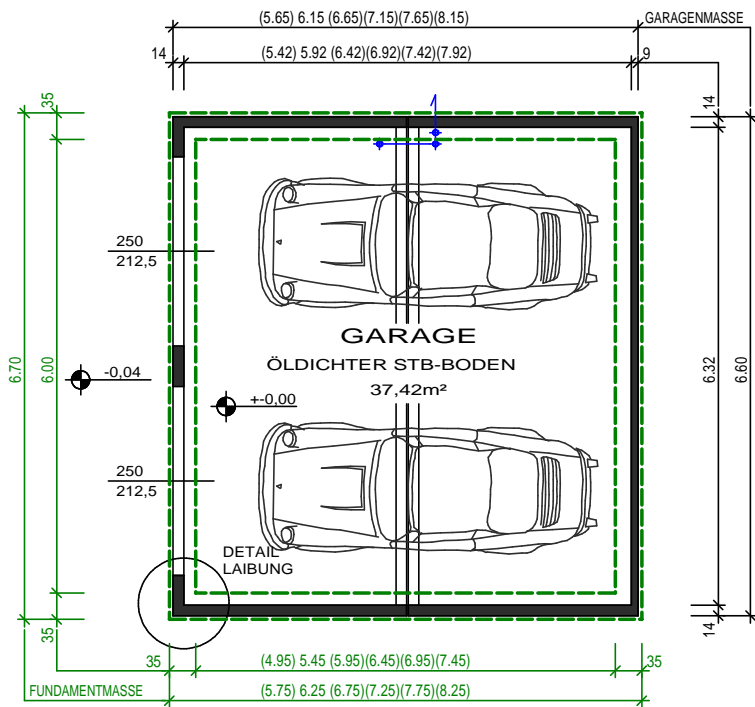
GRUNDRISS
