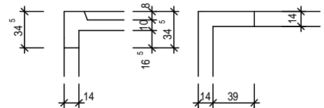
DETAIL STURZ
