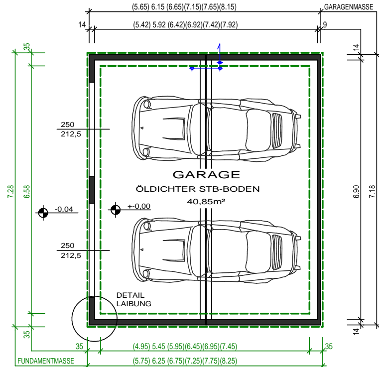
GRUNDRISS
