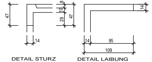
DETAIL STURZ
