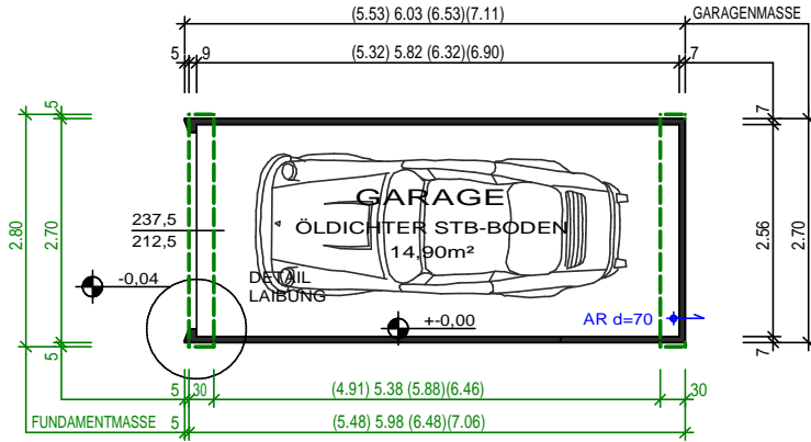
GRUNDRISS
