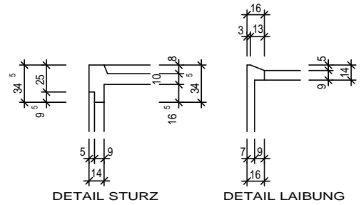
DETAIL STURZ
