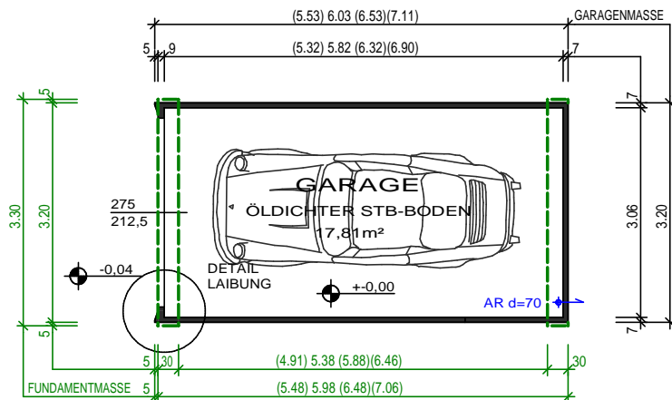
GRUNDRISS
