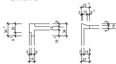
DETAIL STURZ
