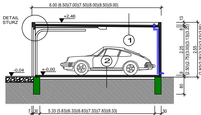
SCHNITT
